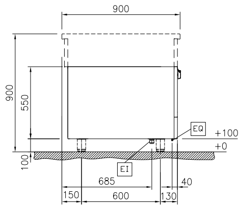
Zij aanzicht
